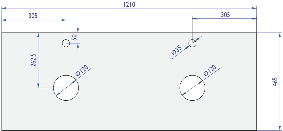
PLAN POUR MEUBLE DE 120 CM
