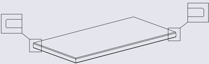
ANGOLARE BORDO COSTA DX/SX 40x80 - 16"x31,5" GRIP RETT.
