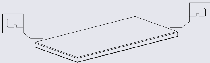
ANGOLARE BORDO COSTA CON GOCCIOLATOIO DX/SX 50x100 - 20"x40" GRIP RETT.
