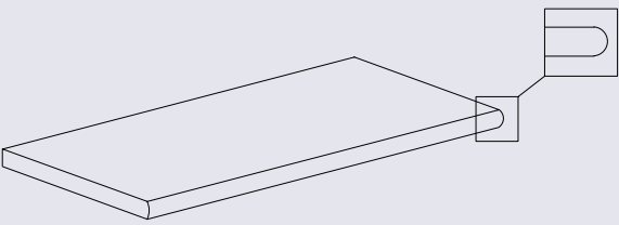
GRADONE CON TORO 40x80 - 16"x31,5" GRIP RETT.
