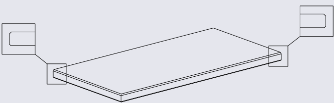
ANGOLARE BORDO COSTA DX/SX 50x100 - 20"x40" GRIP RETT.
